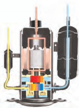
Двоступеневий компресор
