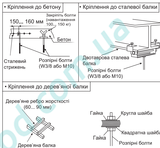
Рис. 3.3.1. Монтаж розпірних болтів
