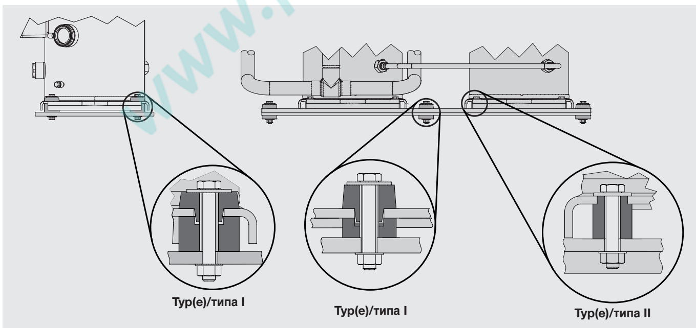
Abb. 2 Schwingungsdämpfer
